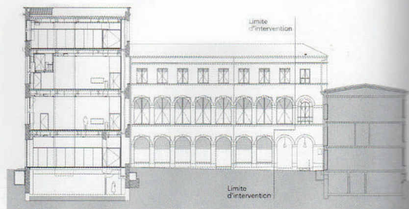
COUPE TRANSVERSALE
